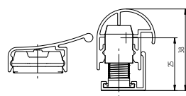
Außenprofil mit Grundprofil
